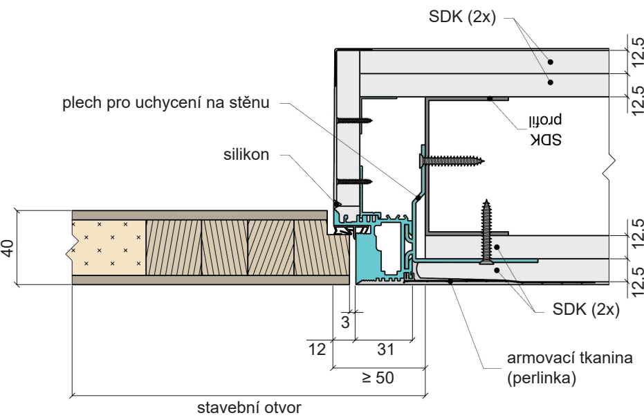
Horizontální řez
