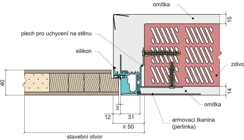
Horizontální řez
